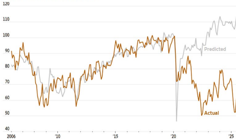
Actual vs. predicted consumer sentiment
